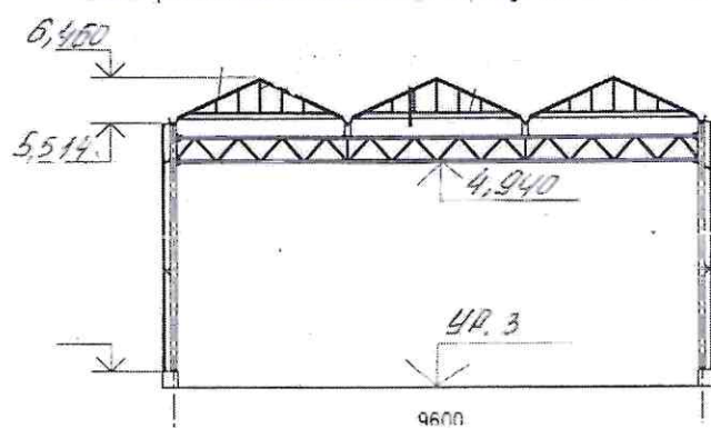
Схема расположения элементов ограждения Участок № 6
