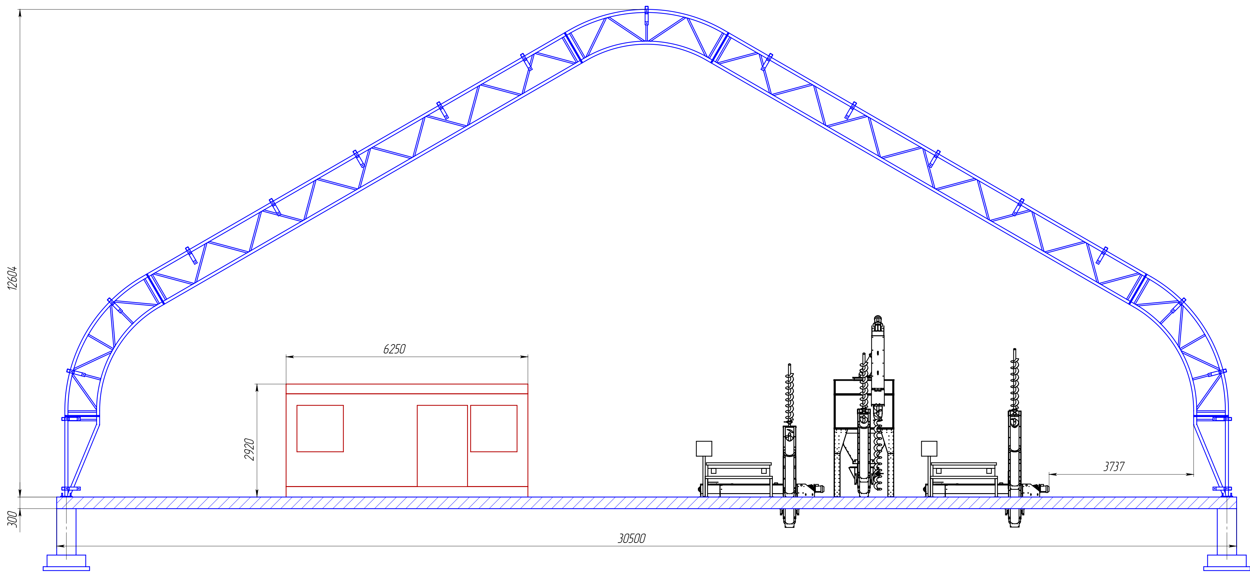
Б-Б (1 : 60)
