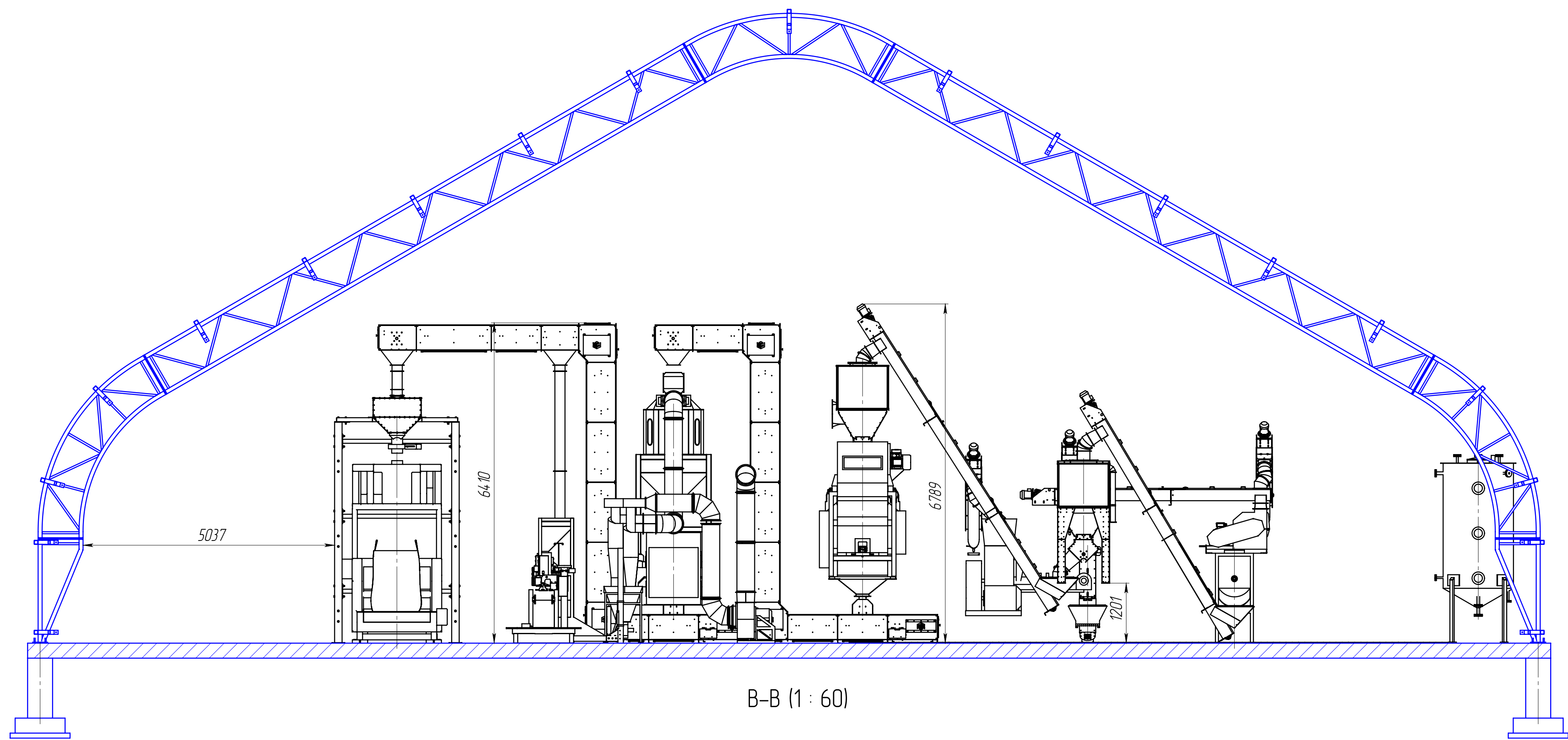
Б-Б (1 : 60)
